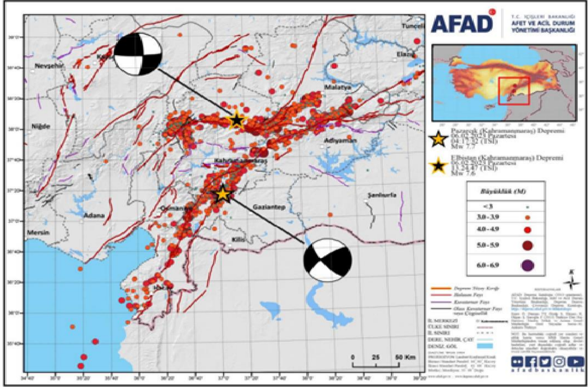
06.02.2023 Pazarlık (Kahramanmaraş) Mw7,7 ve Elbistan (Kahramanmaraş) Mw7,6 depremleri ve artçı şok aktivitesi (AFAD)
