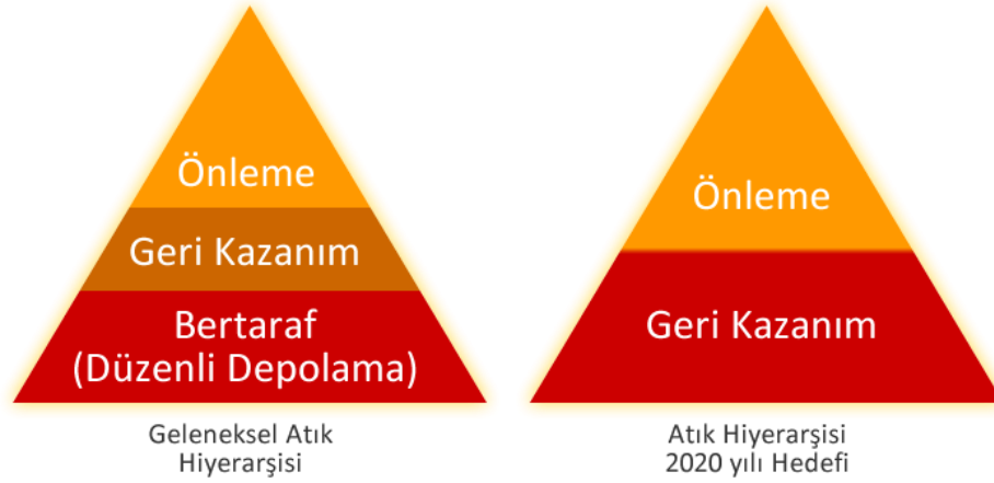
Şekil 2.1 Konvansiyonel atık bertaraf hiyerarşisi ve 2020 yılı için hedeflenen hiyerarşi
